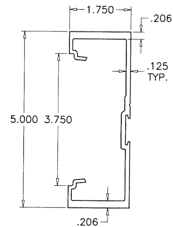
T7 TRANSOM JAMB S-8000
