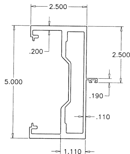
E3 DOOR JAMB Series 9000
