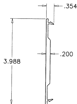
E15 JAMB FILLER
