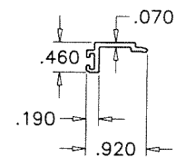
E21 DOOR STOP
