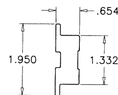
E11 CORNER PLATE
