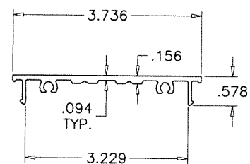
T8 JAMB FILLER S-8000
