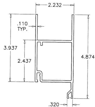
E4 TOP RAIL
